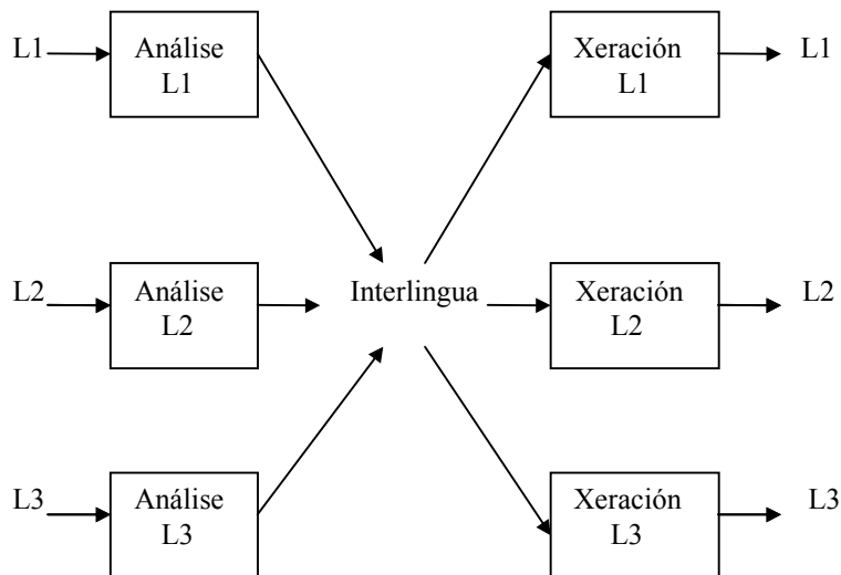
Figura 23. Estratexia de traducción mediante interlingua.
