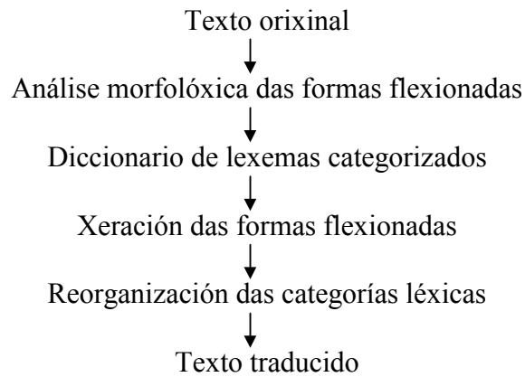
Figura 22. Estratexia de traducción directa ampliada.
