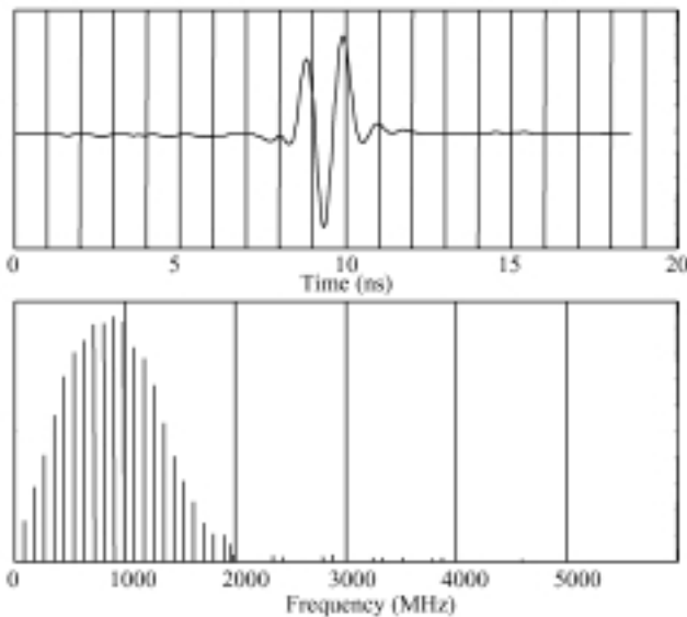
Fig. 1. Forma de la señal (arriba) y espectro (abajo) del impulso generado por una antena de radar de 900 MHz.
