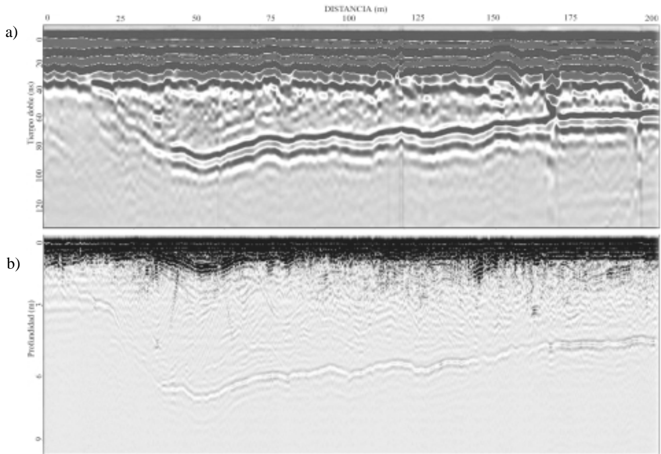
Fig. 8. Perfiles de 200 m efectuados con una antena no apantallada de 100 MHz (a) y otra apantallada de 250 MHz (b) donde se detectan las reflexiones relacionadas con la roca madre. En ambos casos la ventana de tiempos fue fijada en 120 ns, equivalentes a unos 9 m de profundidad.
